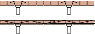
Horizontal section of vertical wall of ICON lattice. Sección horizontal de paramento vertical de celosía ICON.
