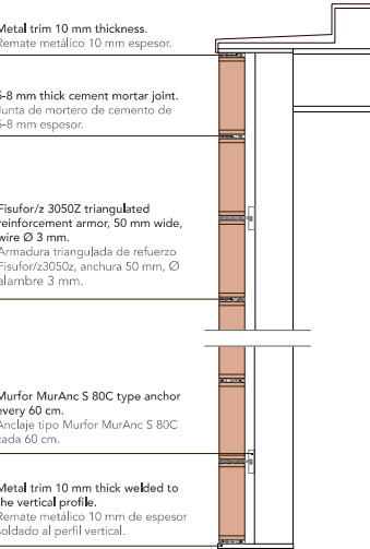
Vertical lattice wall supported by an interior slab. Paramento vertical de celosía apoyado en forjado interior.
